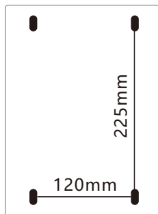
固定孔距离
